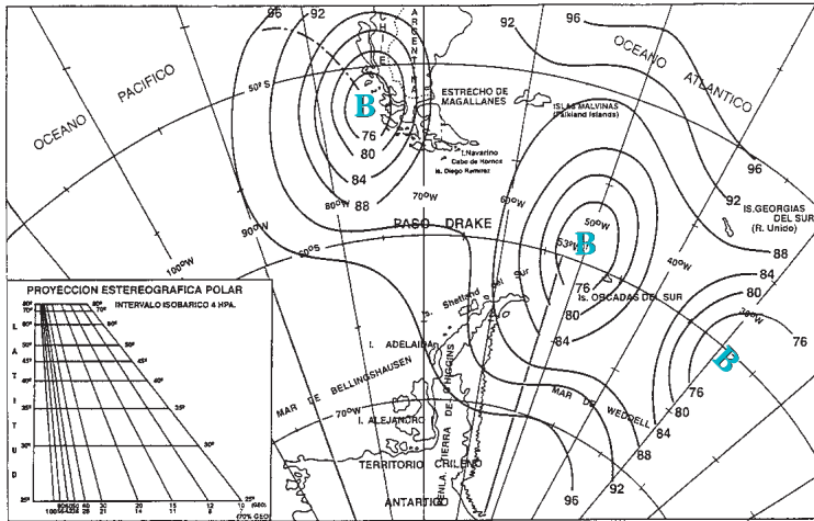
Figura 27. Temporal con viento del Este en Islas Shetland del Sur
